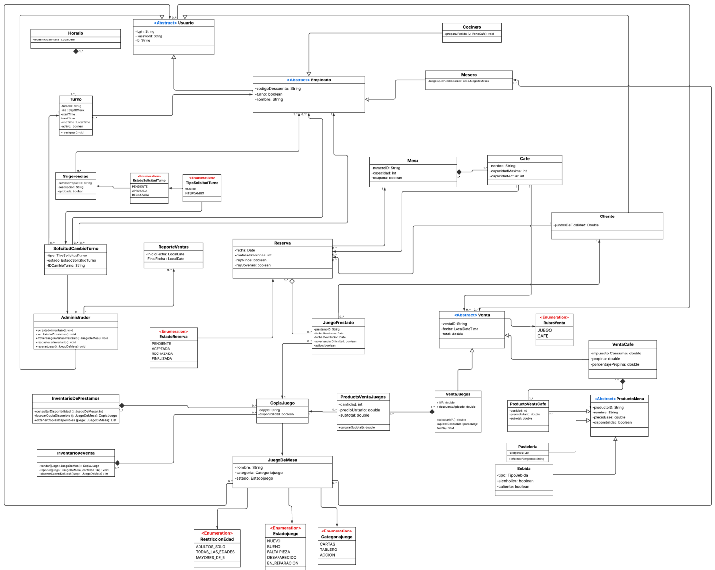
Diagrama de Clases de alto nivel de Board Game Cafe
