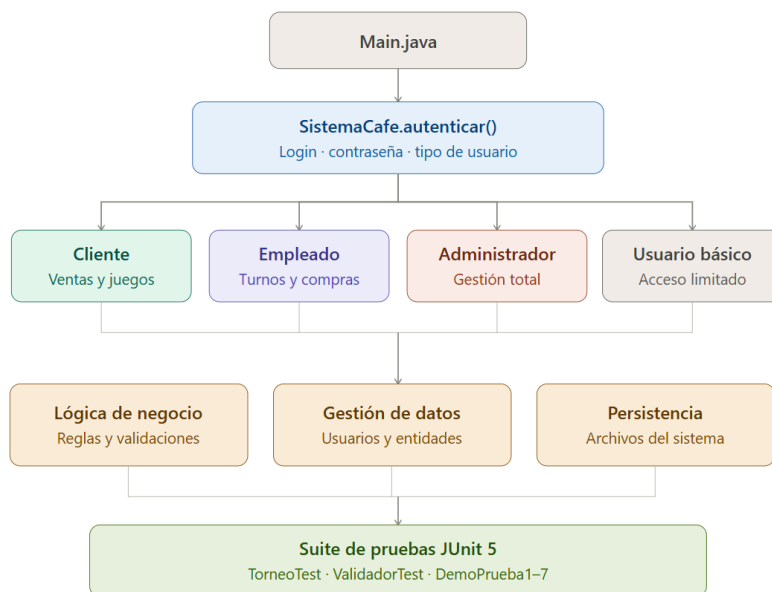
Figura 1. Diagrama de la implementación del BoardGameCafe
